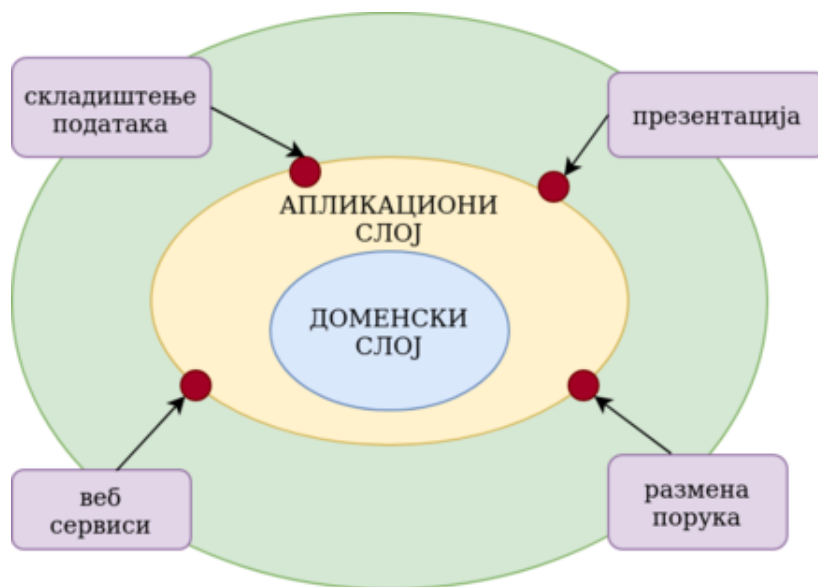
Слика 2.4: Слојевита архитектура апликације са инверзијом зависности
