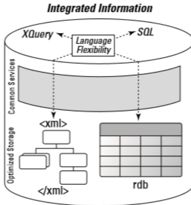
Слика 2.1: pureXML
