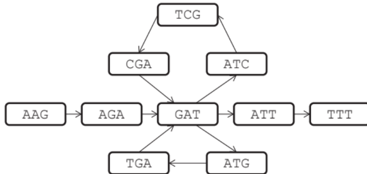
Slika 3.10: De Brojnov graf sa dva ciklusa [12]
