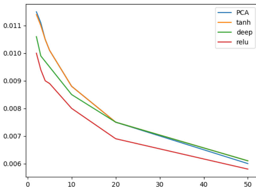
Slika 5.5: Grafik srednje apsolutne greške modela. Na x osi se nalazi dimenzionalnost skrivene reprezentacije, dok se na y osi nalazi srednja apsolutna greška.
