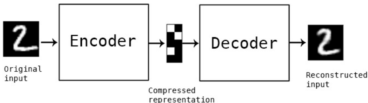
Slika 3.2: Shema autoenkodera na primeru ulaza iz MNIST skupa [3]
