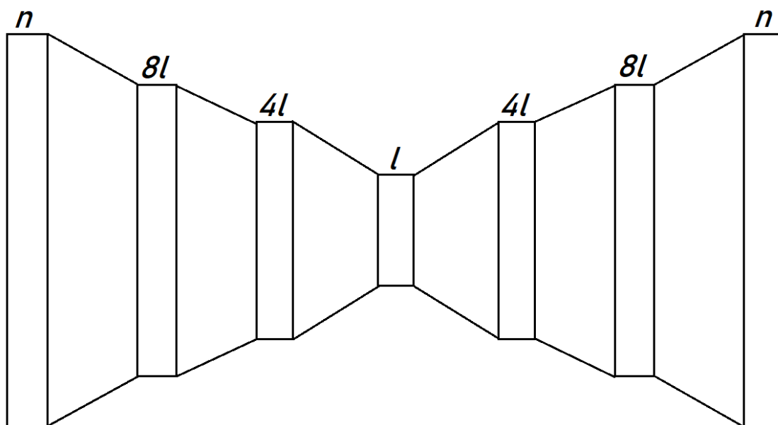
Slika 5.4: Shema dubokog autoenkodera. Ulazni i izlazni sloj imaju n vrednosti, gde je n ukupan broj piksela u ulaznoj mapi. Broj neurona u skrivenim slojevima je umnožak broja l , koji uzima vrednosti iz tabele 5.2. Izlaz skrivenog sloja sa l neurona predstavlja skrivenu reprezentaciju ulaza.
