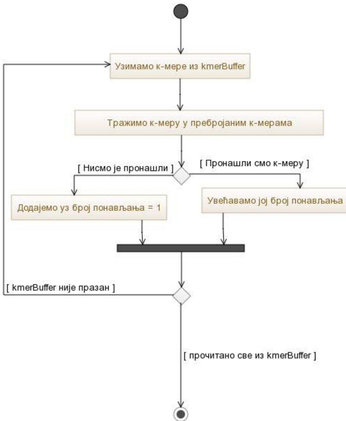
Слика 12. УМЛ Дијаграм активности - Пребројавање к-мера
